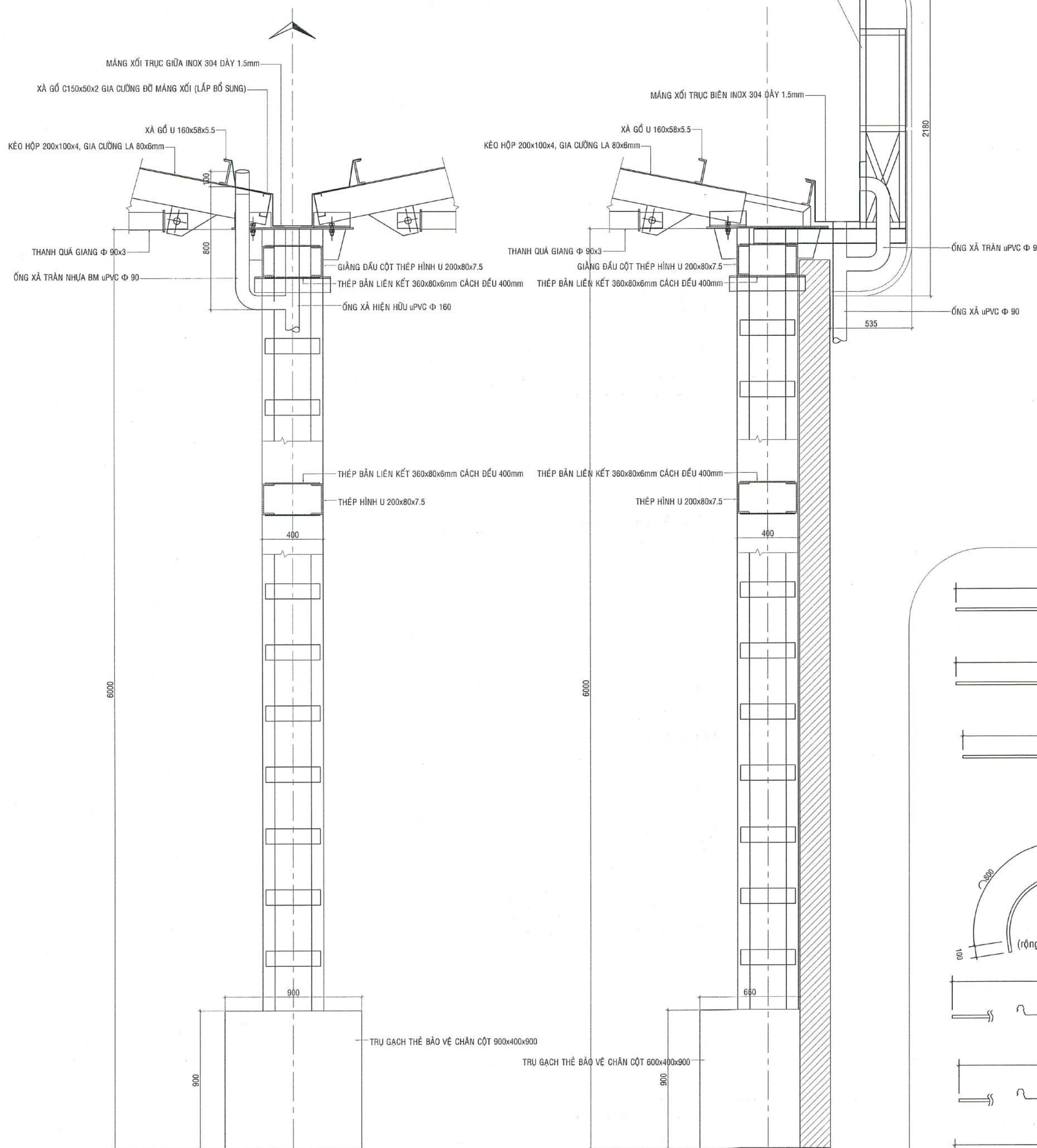
CẤU TẠO CỘT BIÊN VÀ MẶT DỰNG KIẾN TRÚC (60 cây)
